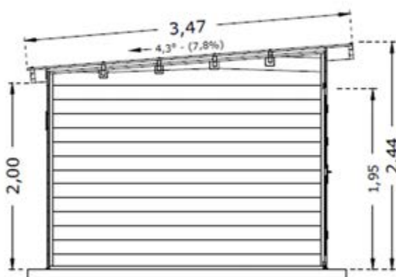
Schnitt / section
