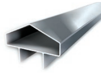
B ABSCHLUSSPROFIL 40x60x1930mm
